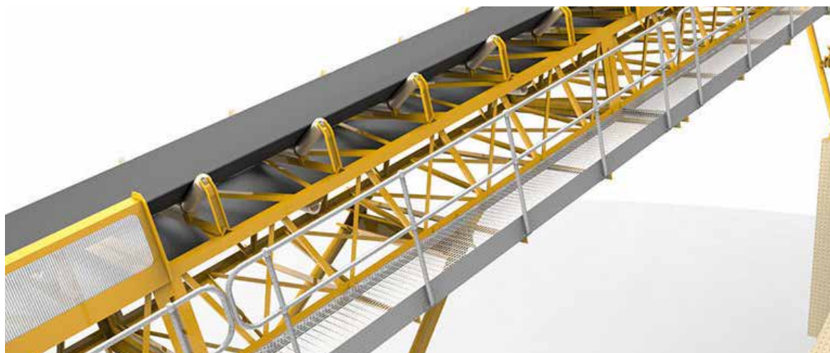
En minería son muy usadas las fajas de tipo Overland, por cubrir una mayor extensión y soportar más carga.
